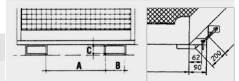
Goupille de sécurité contre tous glissement
