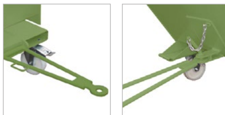
Dispositif d'attelage avec barre de remorquage
