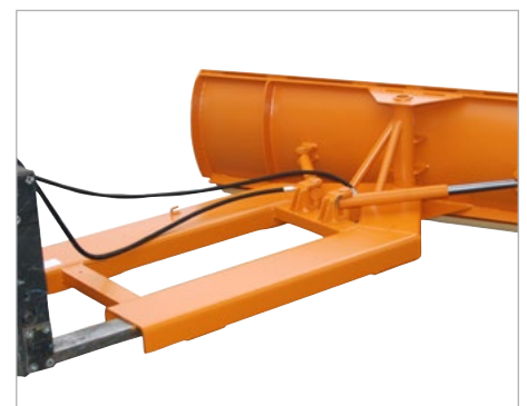
Réglage hydraulique du bouclier
